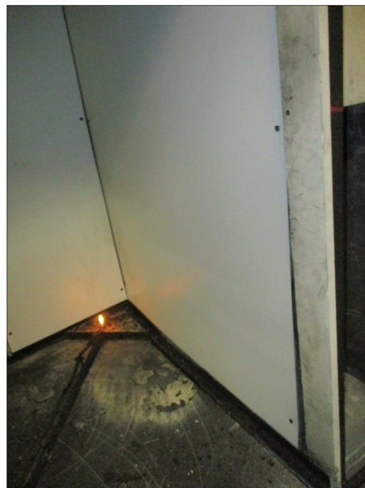
Vista totale del bordo esterno verticale dell'ala lunga prima della prova Total view of the vertical outer edge of the long wing before the test
