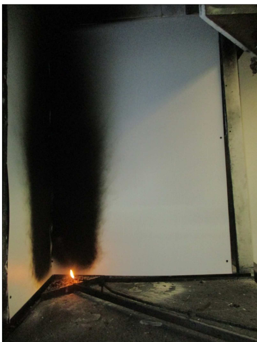
Vista totale della superficie esposta dell'ala lunga dopo la prova Total view of the exposed surface of the long wing after the test
